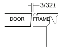
Beaded Inset - BI
